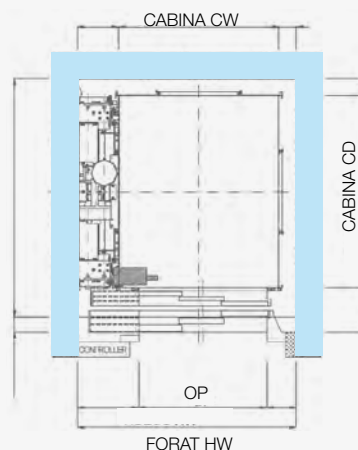
Un embarcament, porta automàtica telescòpica
