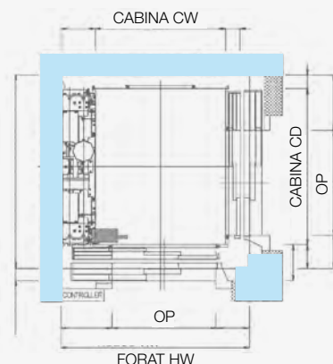
Doble embarcament de 90°, porta automàtica telescòpica
